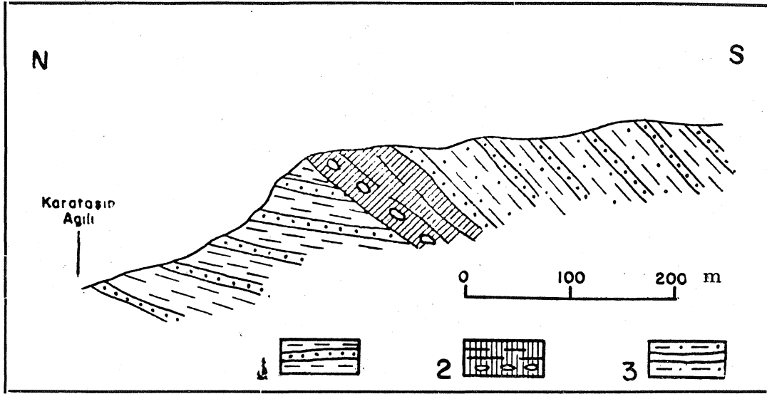
Şek* 2 - Karataşm Ağılı güneyindeki diskordansi gösterir basit bir profil Abb. 2- Vereinfachtes Profil über die Diskordanz südlich von Karataşm Ağılı
