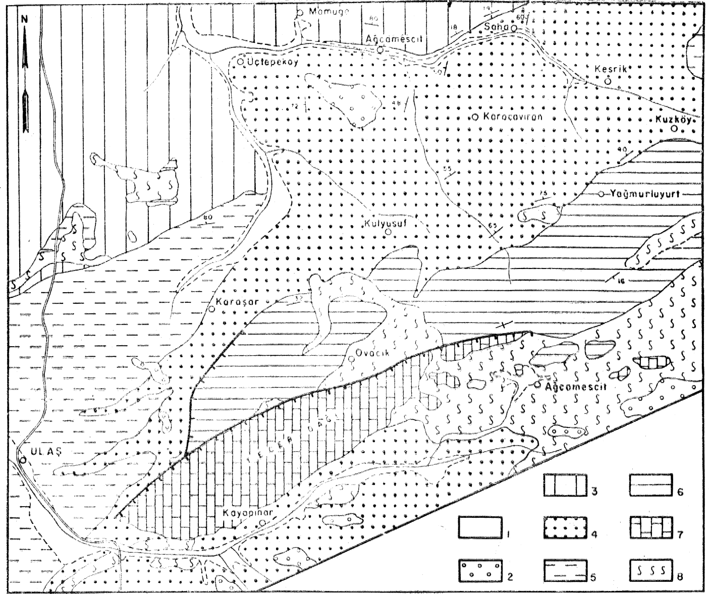
.TECER DAĞLARI BÖLGESİNE AİT JEOLJİK HARİTA GEOLOGISCHE KARTE DES TECERDAĞ-GEBIETES
